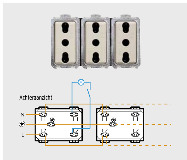
Aansluitschema duplex-triplex stopcontact
